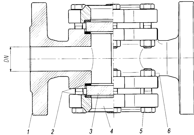
SEZ A-A
