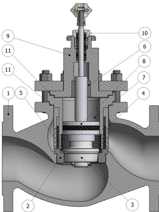
VALVOLA BILANCIATA
