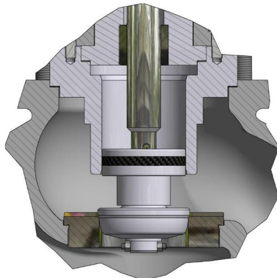
OTTURATORE BILANCIATO
