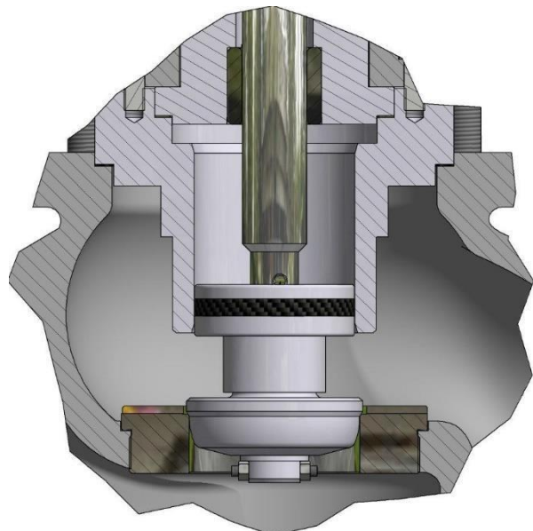
Otturatore bilanciato
